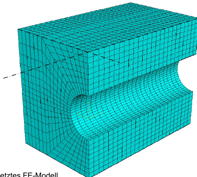
Bild 7-9 Vernetztes FE-Modell
