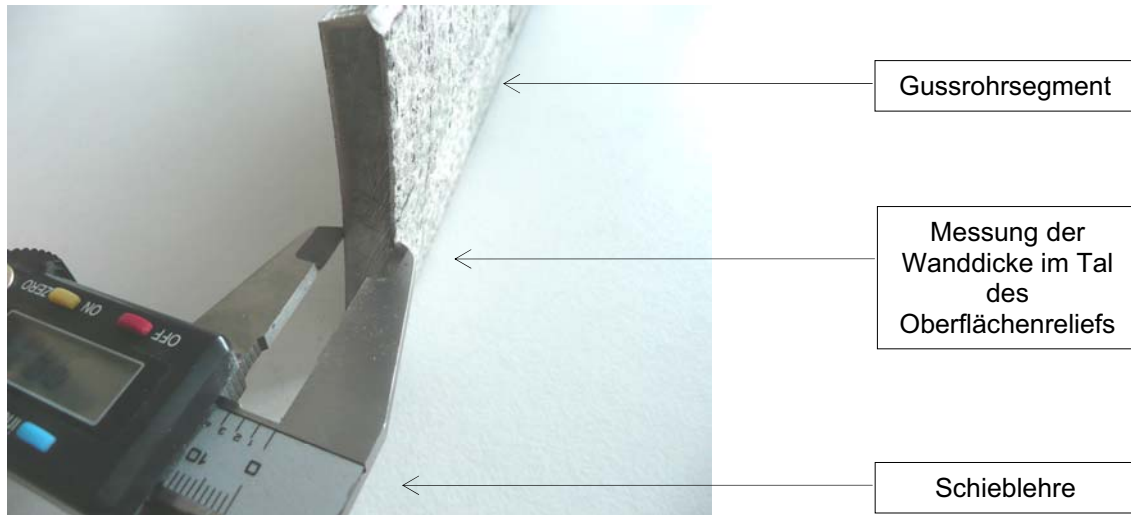
Bild E1-1: Messung der Wanddicke im Tal des Oberflächenreliefs
