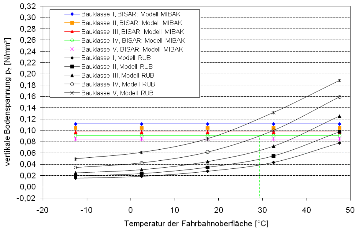
Bild 5-4 Vergleich von vertikalen Bodenspannungen aus [U3] und nach BISSAR 3.0 für eine Stahlplatte in 60 cm Tiefe unter FOK
