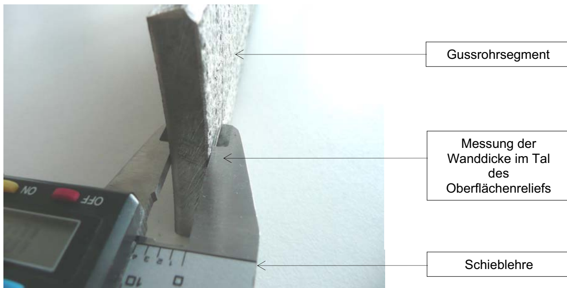
Bild E1-2: Messung der Wanddicke inklusive Wellinger Zone
