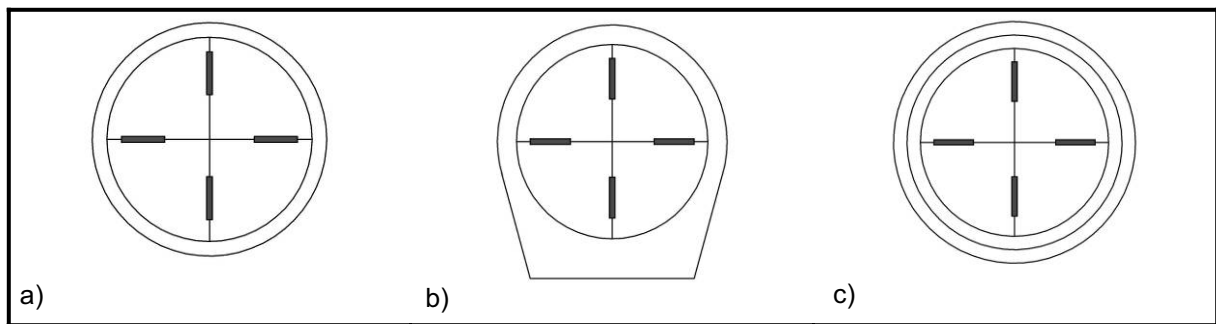
Bild 3-9 Anzahl und Lage der Wegaufnehmer in den Nebenmessquerschnitten a) Guss-, b) Beton- und c) Kunststoff-Rohrstrang
