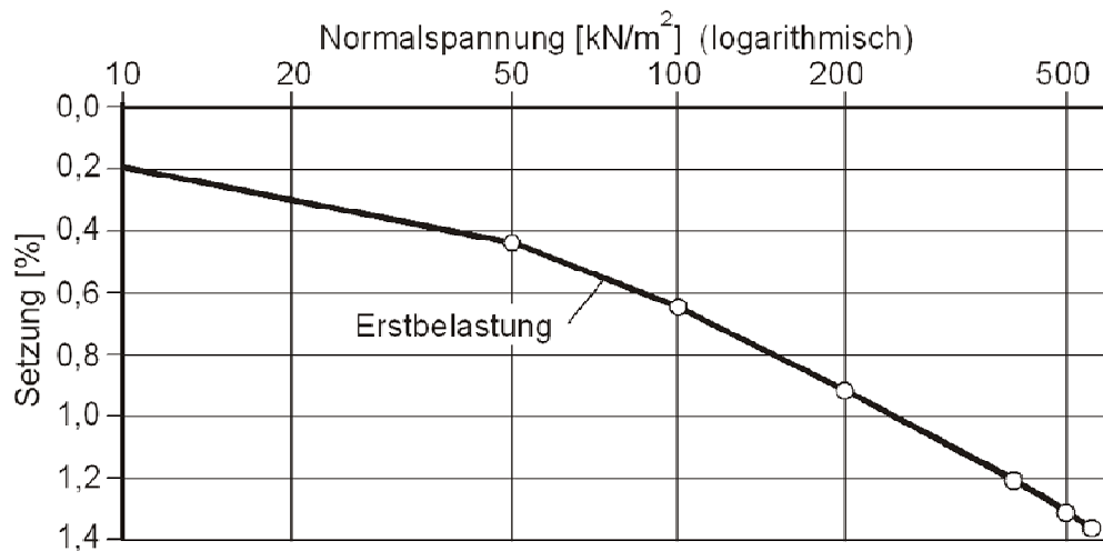
Bild 5-7 Lastsetzungskurve aus Kompressionsversuch für D_{Pr} = 95 \%
