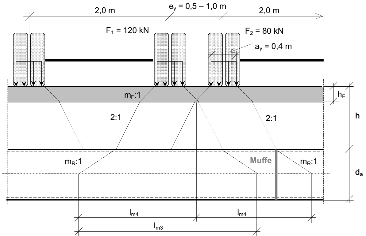
Bild 7-2a Lastverteilung in Rohrlängsrichtung bei Querüberführung, Modell A (maßstäblich für h = 0,88 \text{ m} , h_F = 0,22 \text{ m} )
