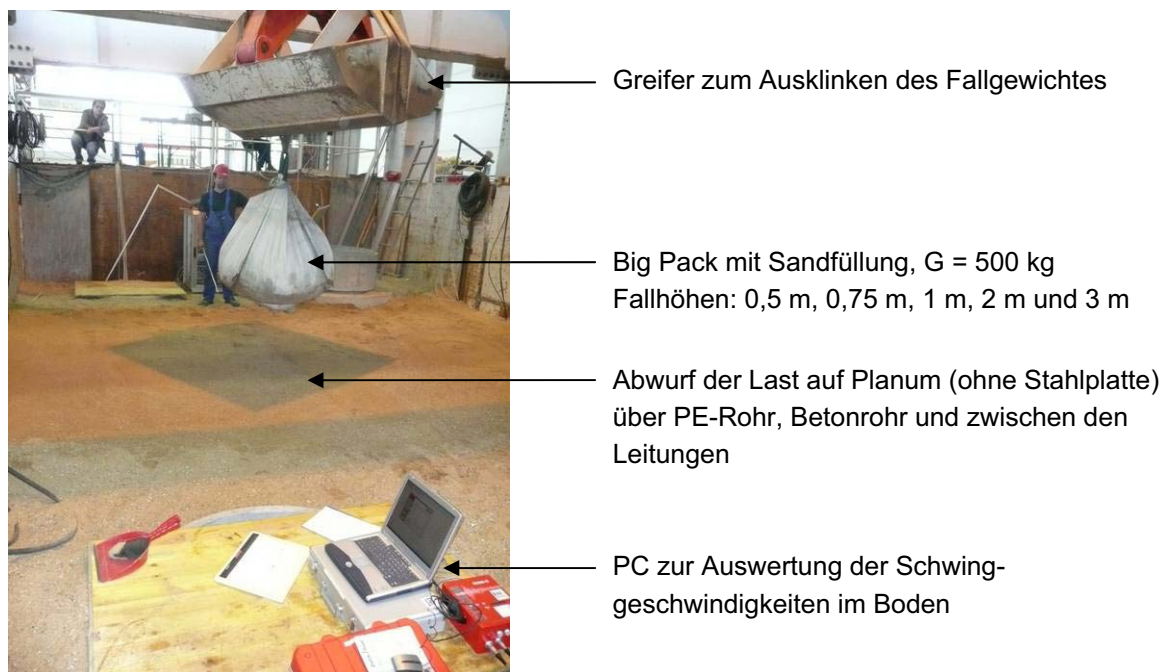
Bild 6-32 Versuchsaufbau für Versuche mit stoßartiger Belastung
