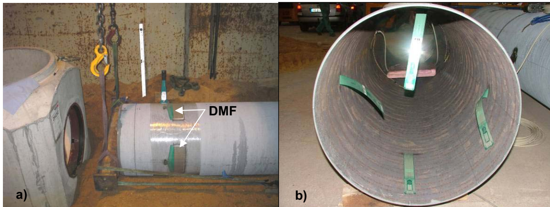
Bild 3-11 Anordnung der Druckmessfolien (DMF) an den Guss-Rohren a) Rohraußen- und b) Rohrinneinnenseite
