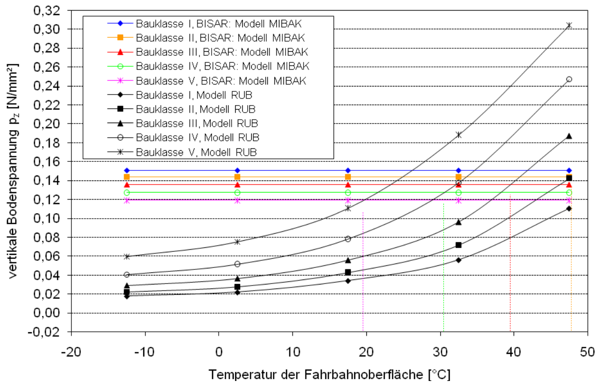
Bild 5-2 Vergleich von vertikalen Bodenspannungen aus [U3] und nach BISSAR 3.0 für eine Stahlplatte in 40 cm Tiefe unter FOK
