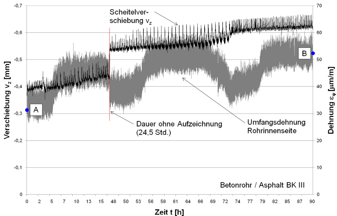
Bild 6-7 Verlauf der Verschiebung und der Umfangsdehnung im Scheitel des Betonrohres bei zyklischer Belastung auf Stahlplatten (Simulation Asphalt BK III nach [V8]) A: \varepsilon_\phi bei N = 0 , B: \varepsilon_\phi = bei N = 10^6 (Abschluss der Lastzyklen)
