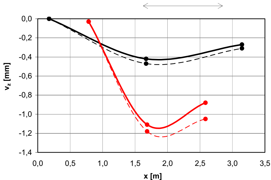
Bild 6-23 Verlauf der Rohrverformungen in Längsrichtung bei normaler Laststellung (NL), für Fahrbahnen der Bauklassen III und V, Markierung = Position der Wegaufnehmer (Rohranfang: x = 0 , Rohrende: x = 3,55 \text{ m} ) Überdeckung BK III: h = 0,88 \text{ m} , BK V: h = 0,80 \text{ m} , vgl. Anhang B44 (Guss) und B83 (PE)
