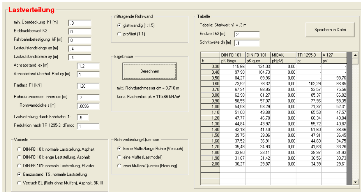
Bild 7-3b Bodenspannung für den Bauzustand, keine Befestigung der Oberfläche (BZ)
