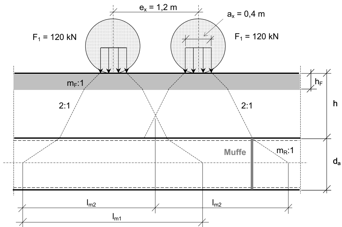
Bild 7-1a Lastverteilung in Rohrlängsrichtung bei Längsüberfahung, Modell A (maßstäblich für h = 0,88 \text{ m} , h_F = 0,22 \text{ m} )
