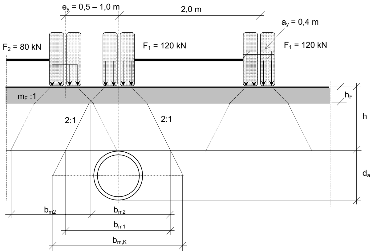
Bild 7-1b Lastverteilung quer zur Rohrleitung mit Begegnungsverkehr bei Längsüberfahung, Modell A
