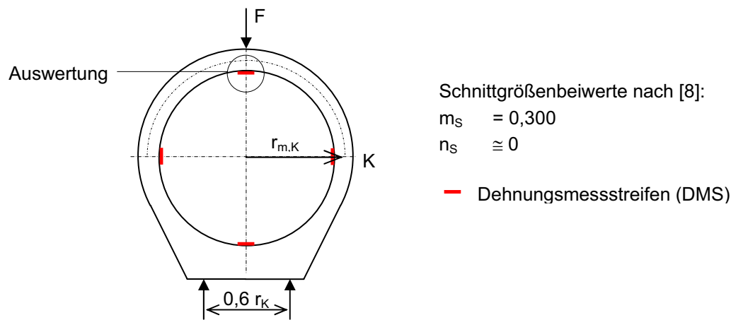
Bild 4-3 Lagerungsfall 2 mit zugehörigen Schnittgrößenbeiwerten nach [8], Anordnung der DMS
