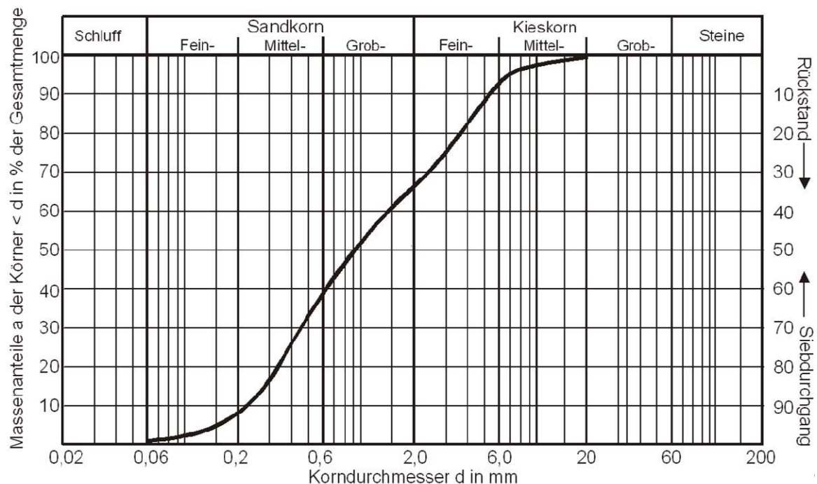
Bild 5-5 Korngrößenverteilung
