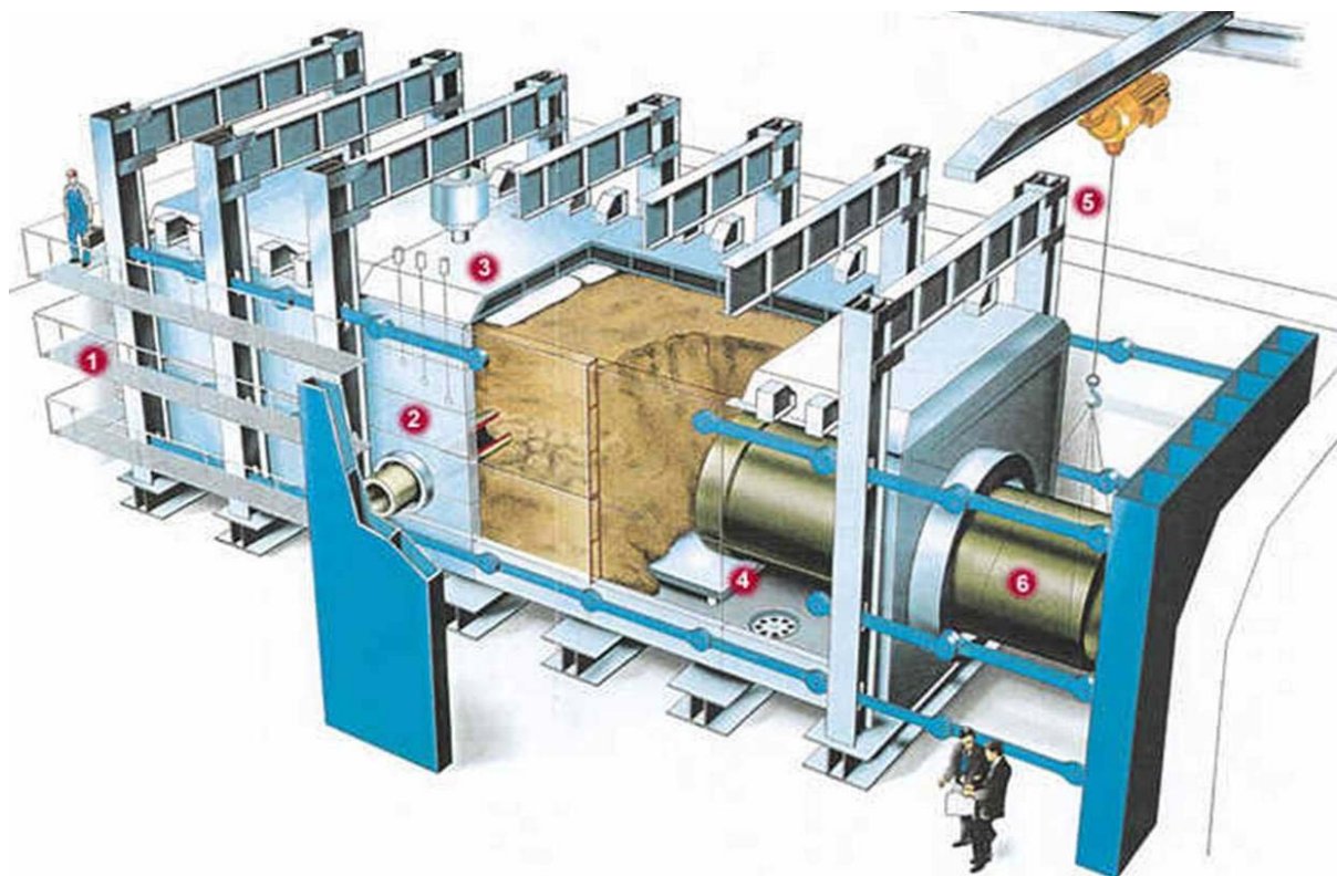
Bild 3-1 Systemskizze IKT-Großversuchsstand
