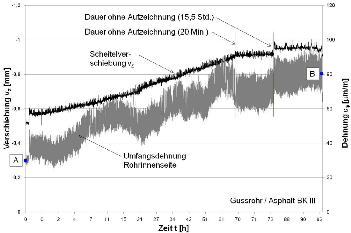
Bild 6-6 Verlauf der Verschiebung und der Umfangsdehnung im Scheitel des Gussrohres bei zyklischer Belastung auf Stahlplatten (Simulation Asphalt BK III nach [V8]) A: \varepsilon_\phi bei N = 0 , B: \varepsilon_\phi = bei N = 10^6 (Abschluss der Lastzyklen)
