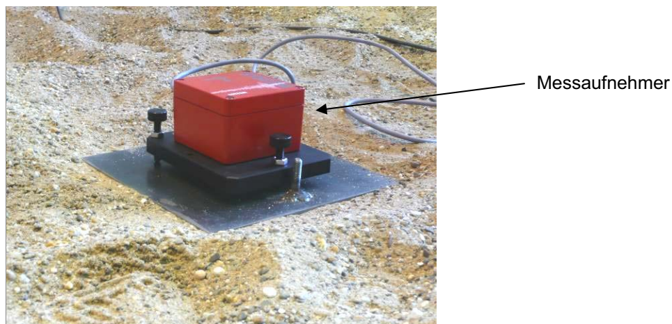
Bild 6-33 Messaufnehmer für Schwinggeschwindigkeiten in x-, y- und z-Richtung
