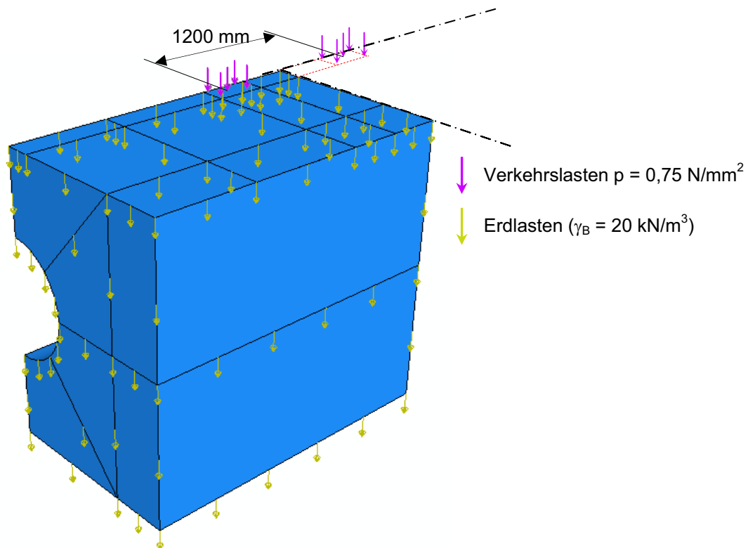
Bild 7-12 Radlasten / Bodenlasten (Darstellung zur Verdeutlichung der Lasten um 180^\circ gedreht)
