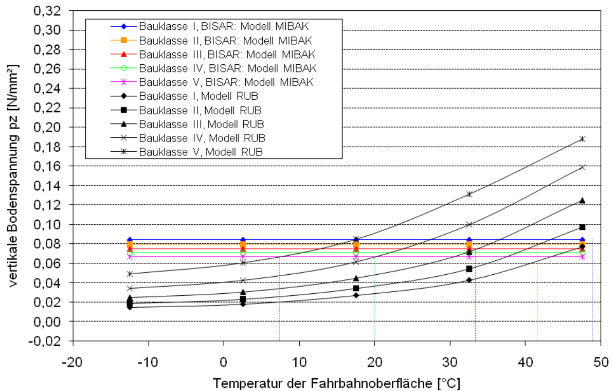
Bild 5-3 Vergleich von vertikalen Bodenspannungen aus [U3] und nach BISSAR 3.0 für zwei Stahlplatten in 60 cm Tiefe unter FOK
