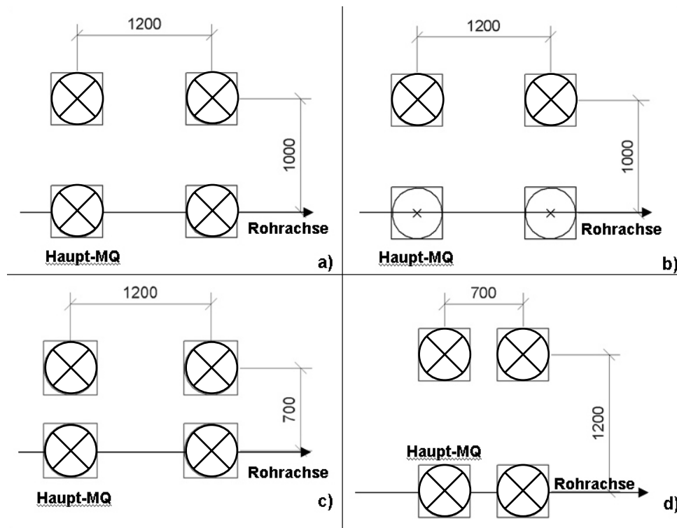
Bild 3-14 Laststellungen beim Lastfall „Radgruppe statisch“
