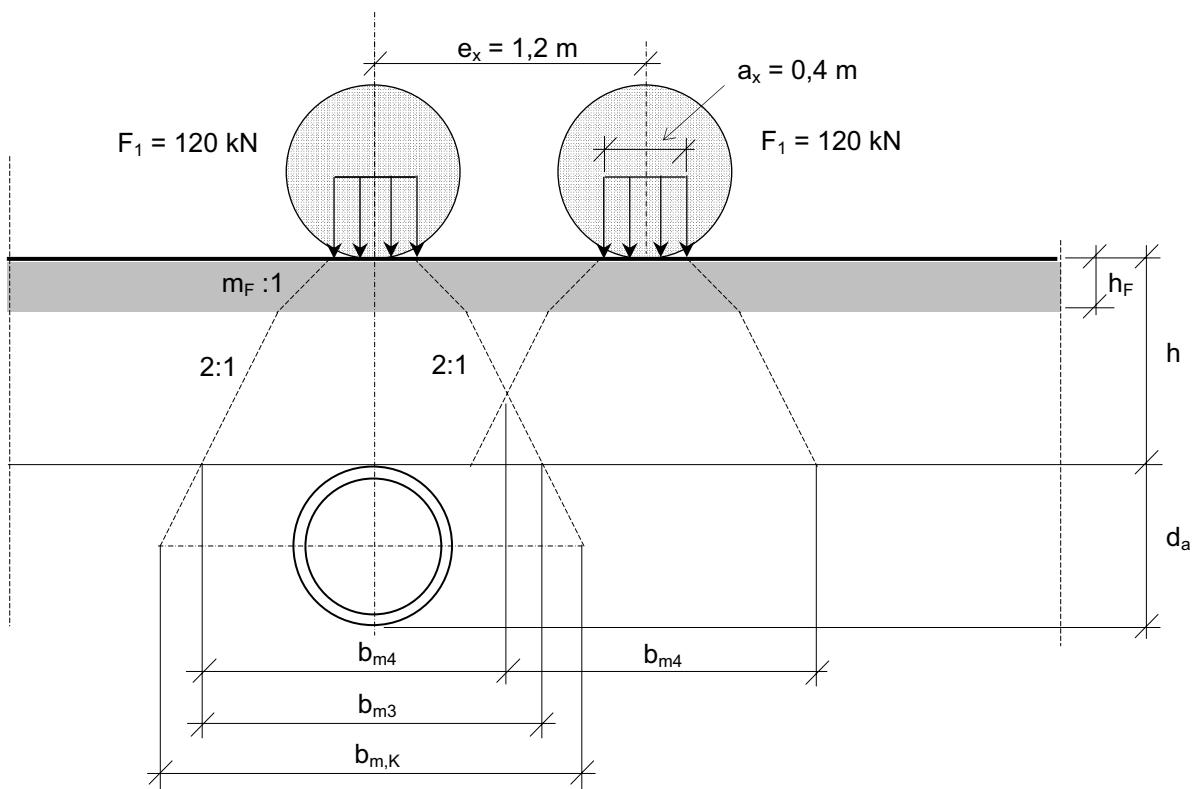
Bild 7-2b Lastverteilung quer zur Rohrleitung mit Begegnungsverkehr bei Querüberführung, Modell A
