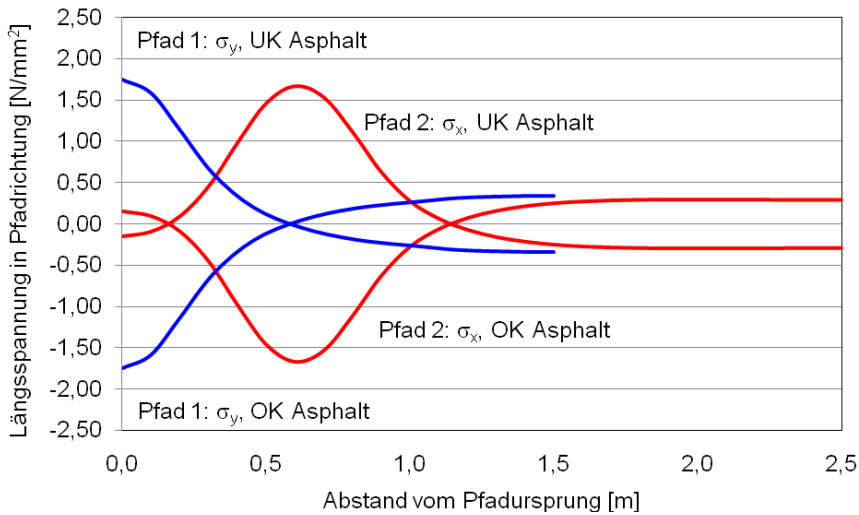
Bild 6-18 Fahrbahnspannungen für das Modell mit einem Betonrohr
