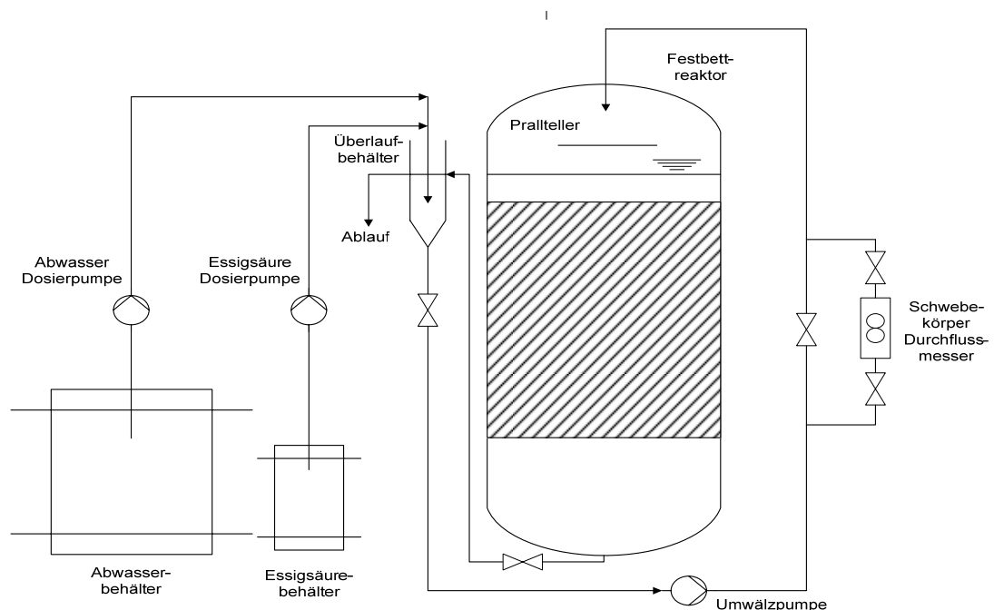
Verfahrensschema der Versuchsanlage zur Denitrifikation in Steinfurt
