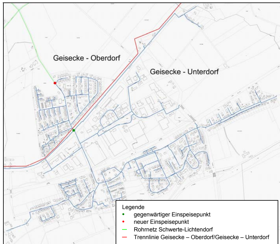
Rohrnetz Geisecke
